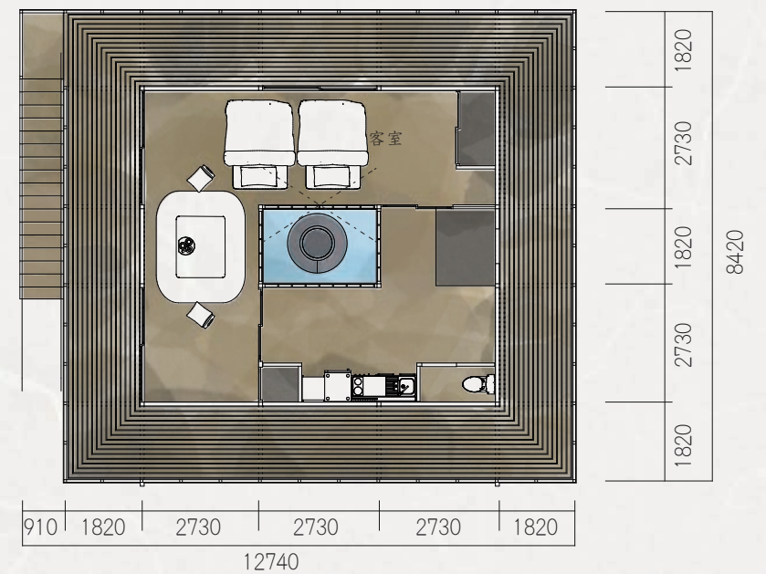
2階平面図
