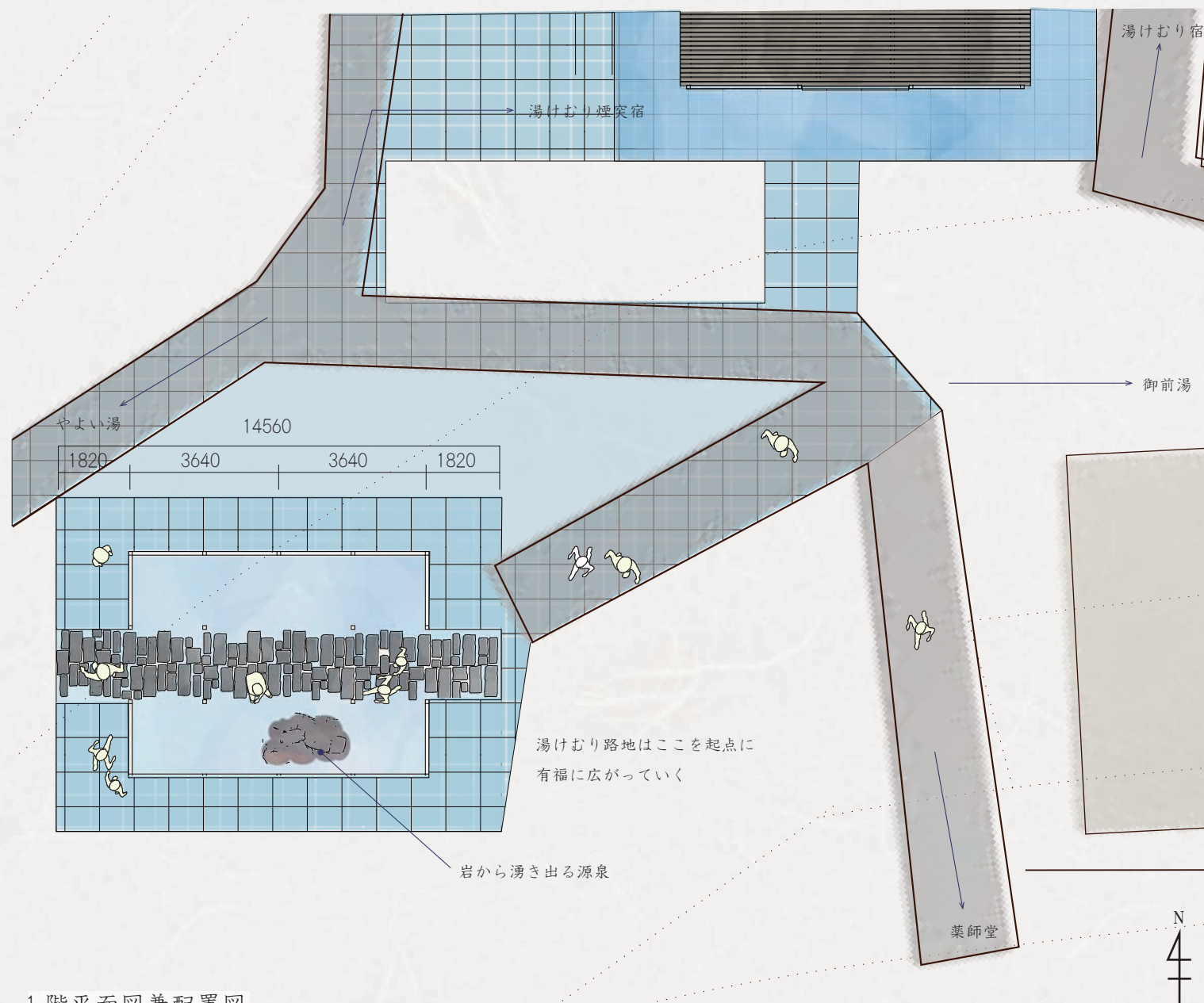
1 階平面図兼配置図
